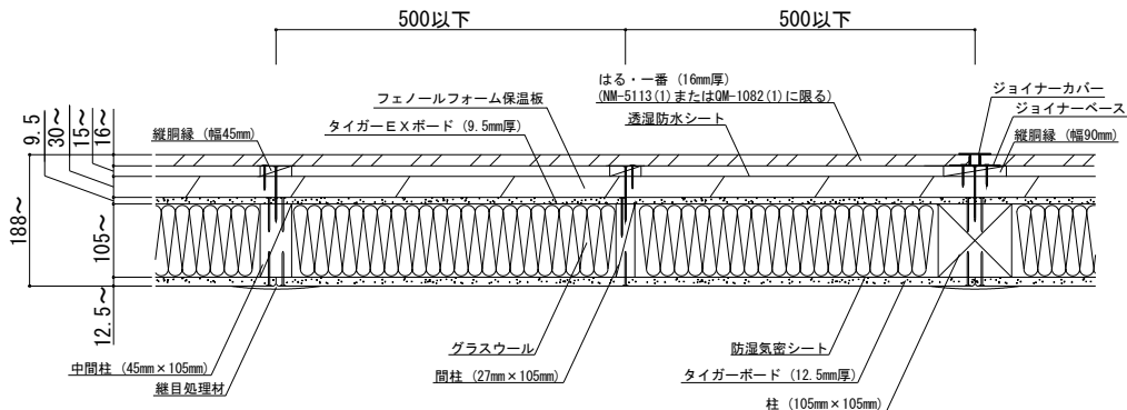
【はる・一番縦張り (横胴縁) 仕様】 (中空部に断熱材を挿入した場合の壁構造)
