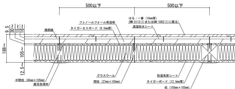
【はる・一番縦張り (横胴縁) 仕様】 (中空部に断熱材を挿入した場合の壁構造)
